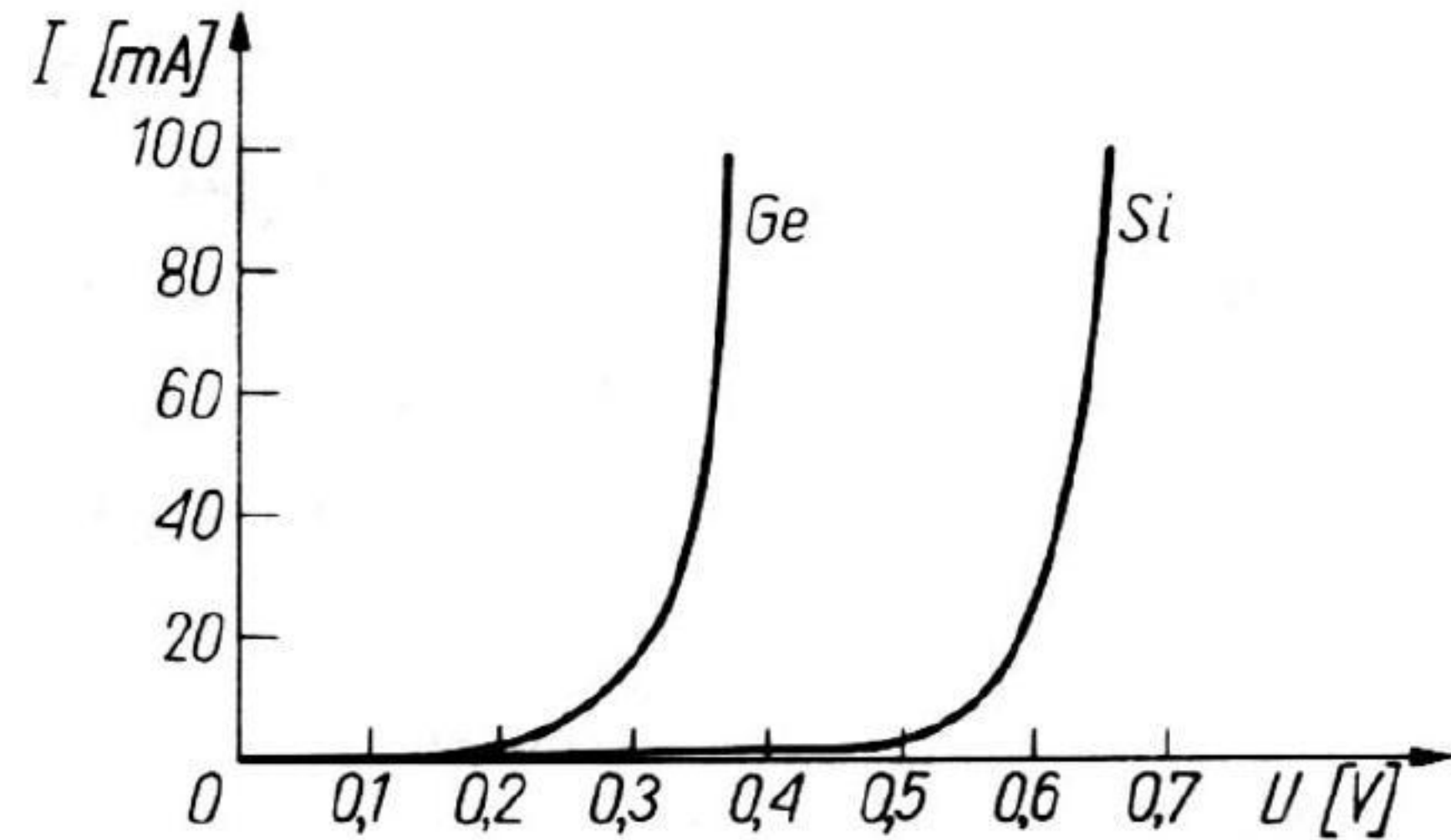
Rys. 2. Charakterystyki I - U diody germanowej i krzemowej przy polaryzacji przewodzenia
